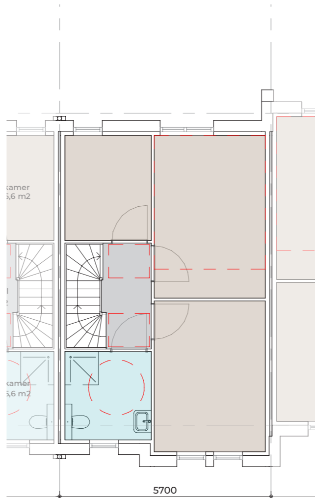
1 e verdieping
