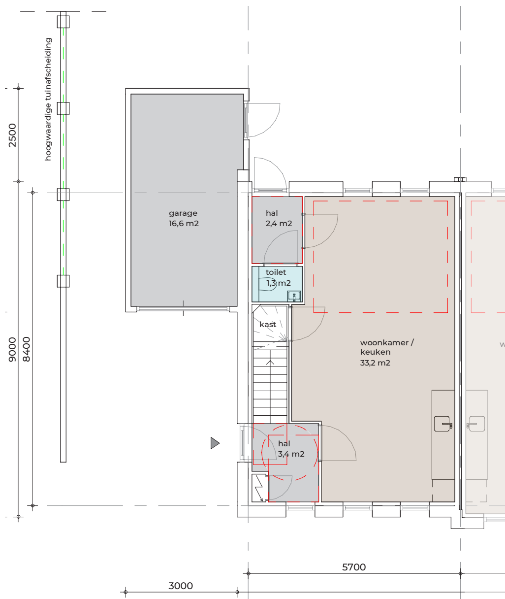
begane grond
