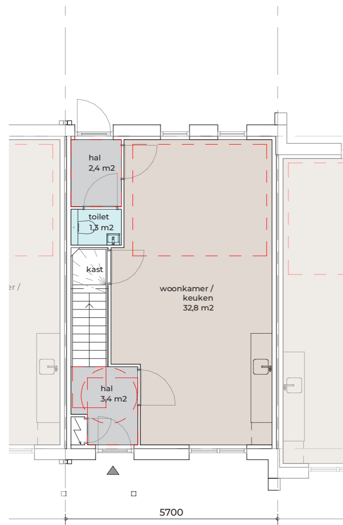
begane grond
