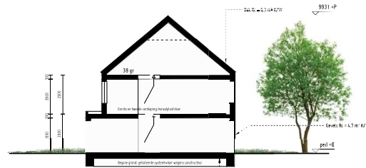
DOORSNEDE
