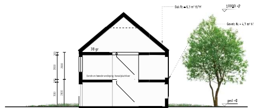
DOORSNEDE
