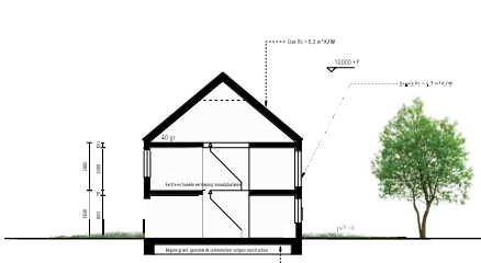
DOORSNEDE
