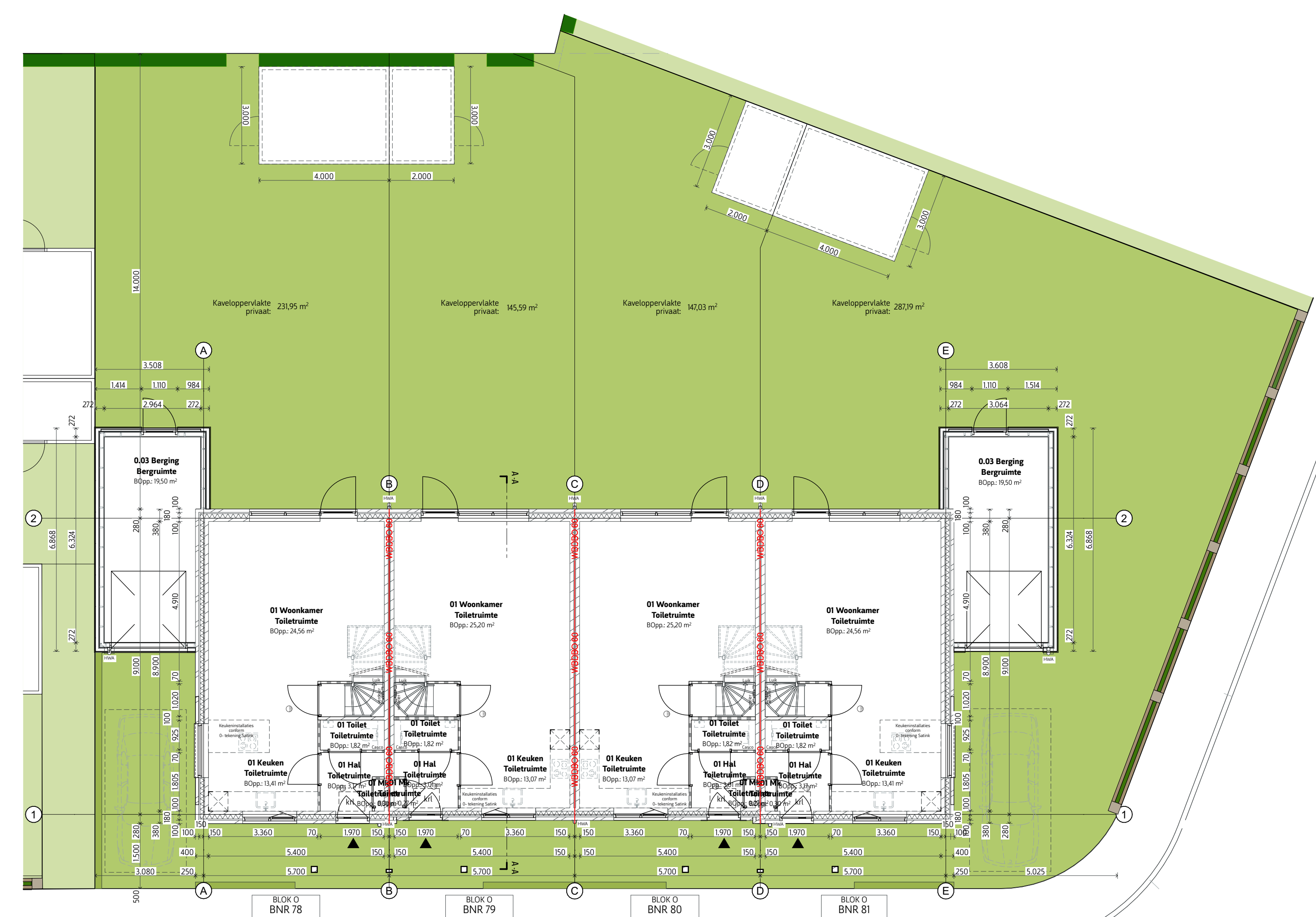
BEGANE GROND #48 t/m #51
