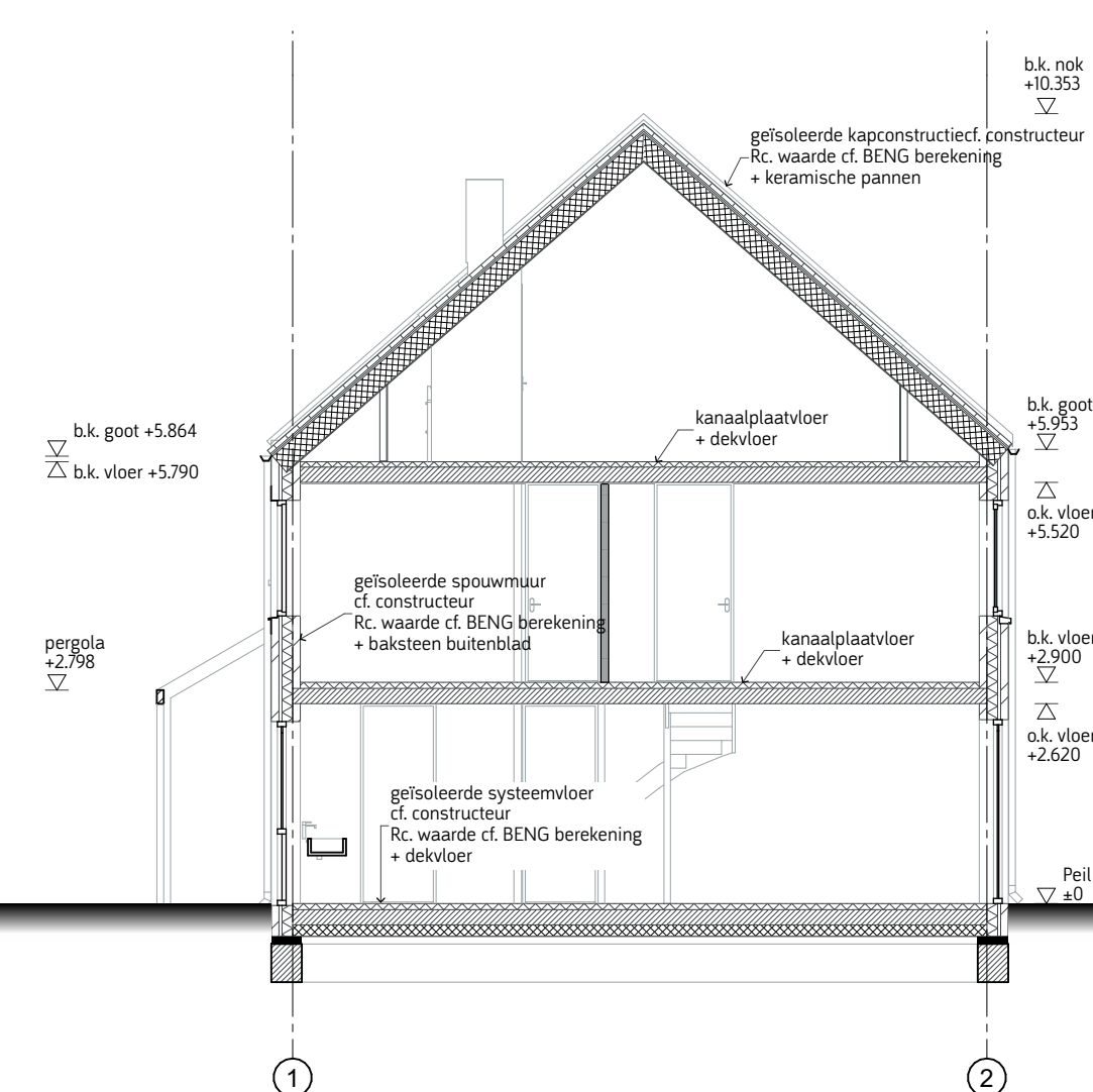
DOORSNED E RIJWONING A-A
