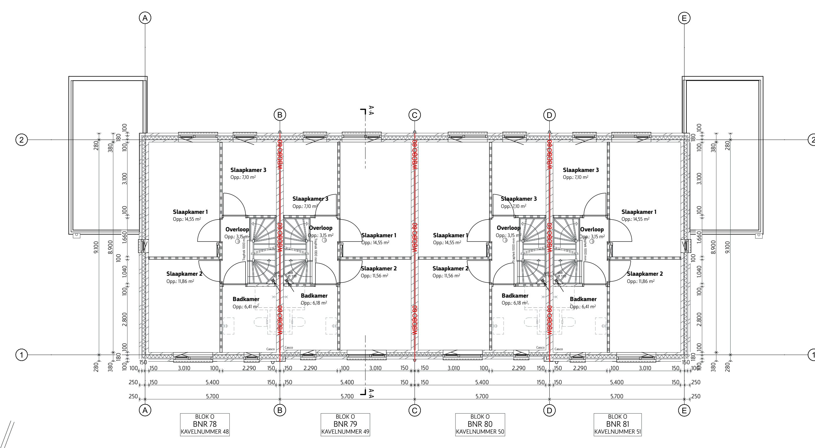
1e VERDIEPING #48 t/m #51
